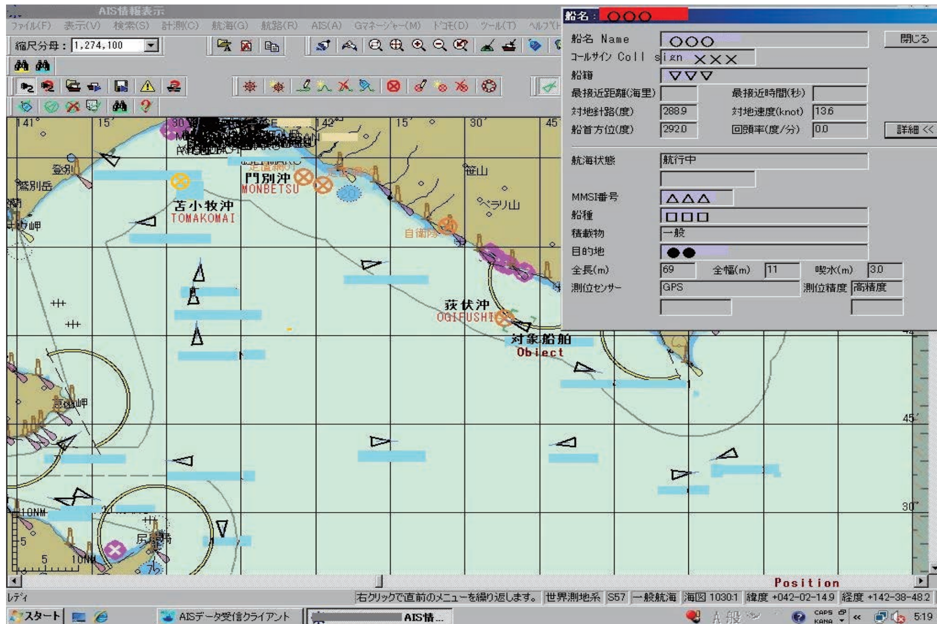
別紙 A I S 端末のパソコン画像 (画像の右上欄は対象船舶の状況)
